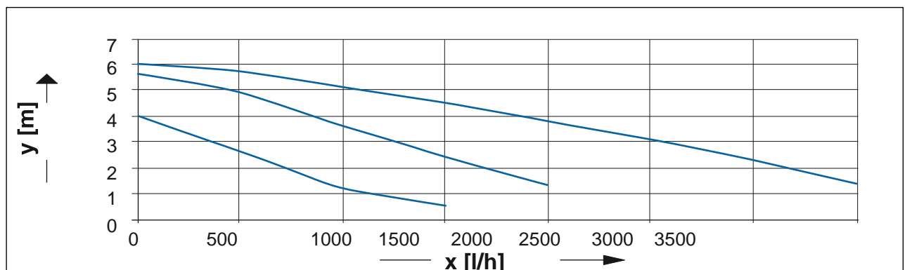
Рис. 8 Напір насоса на прикладі Wilo RS15/6
