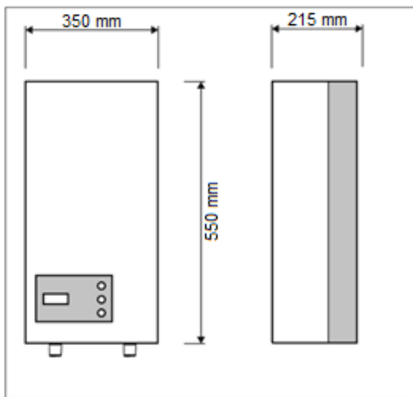
Рис. 2 Розміри опалювального котла AVL Joule AJAX-SPT
