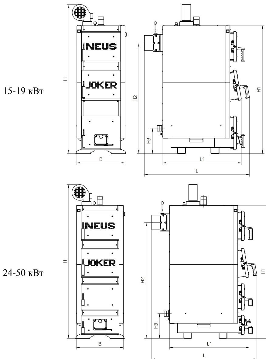
Рисунок 1 – Габаритне креслення котла Неус-Джокер (Неус-Джокер-Плюс)
